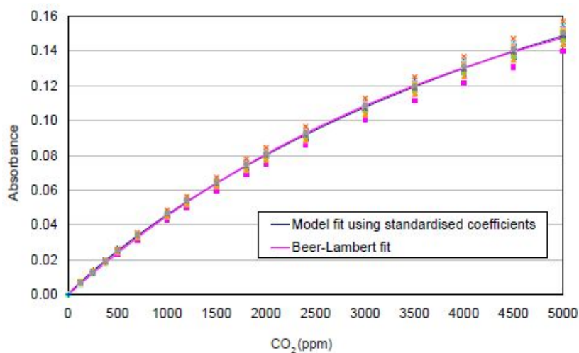
图3 线性度
