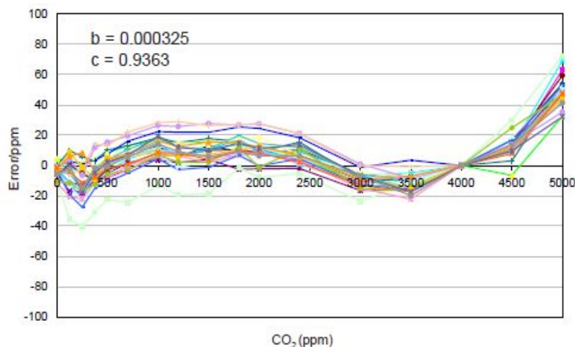
图3 线性度
